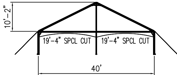
VIEW A-A
