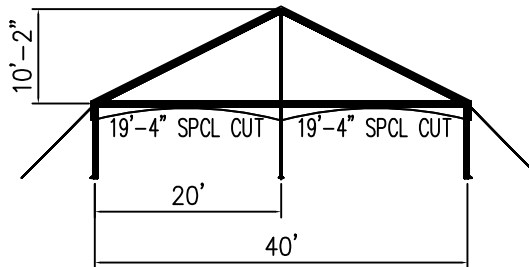
VIEW A-A
