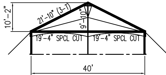
VIEW A-A
