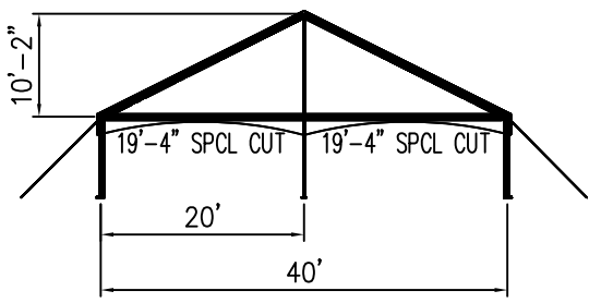
VIEW A-A
