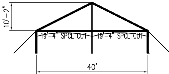
VIEW A-A
