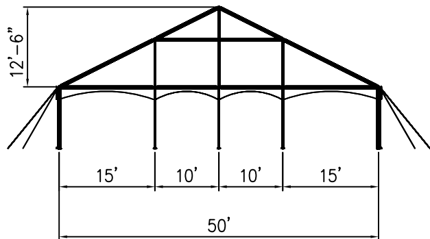
VIEW A-A
