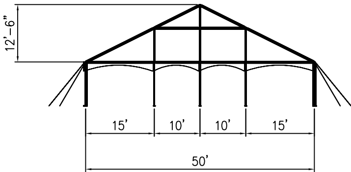
VIEW A-A
